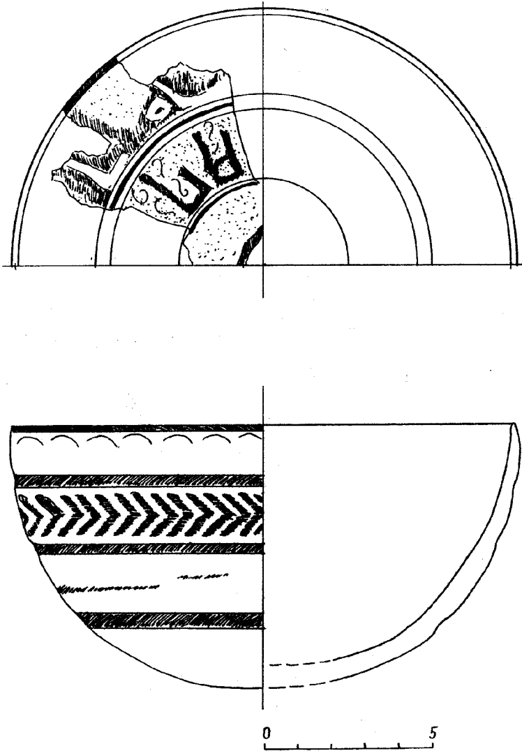
Рис.8. Кашинная чаша с росписью люстром и кобальтом (реконструкция).
